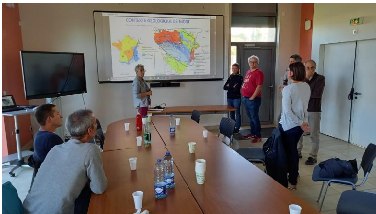
Le contexte géologique et hydrogéologique de la source karstique du Vivier par Hélène
