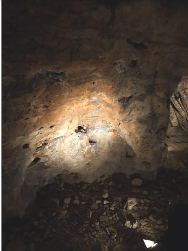
Vue des géodes et détail d'une géode complètement exploitée
